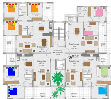
ΚΑΤΟΨΗ 1ου ΟΡΟΦΟΥ
